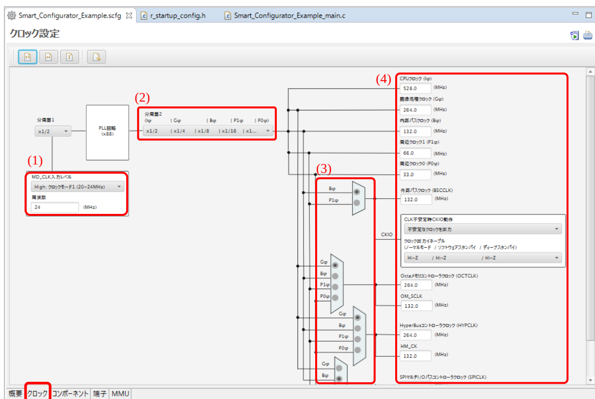
図 4-1 クロック設定
